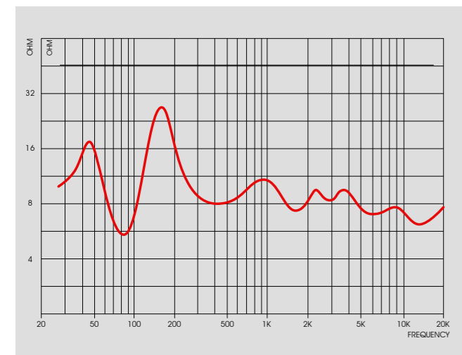
多音路喇叭的阻抗曲線
