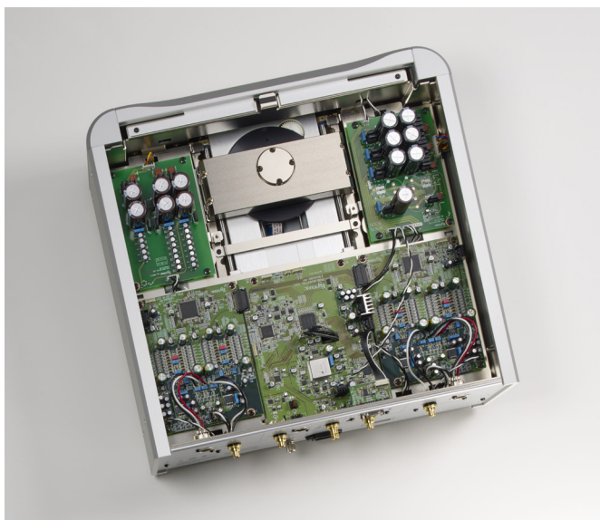
K-01XD的內部還是分為上下二層，上層是VRDS-ALTAS 01讀取系統，以及中央的數位線路板、左右二側的數位類比轉換線路板。圖中就是上層。
