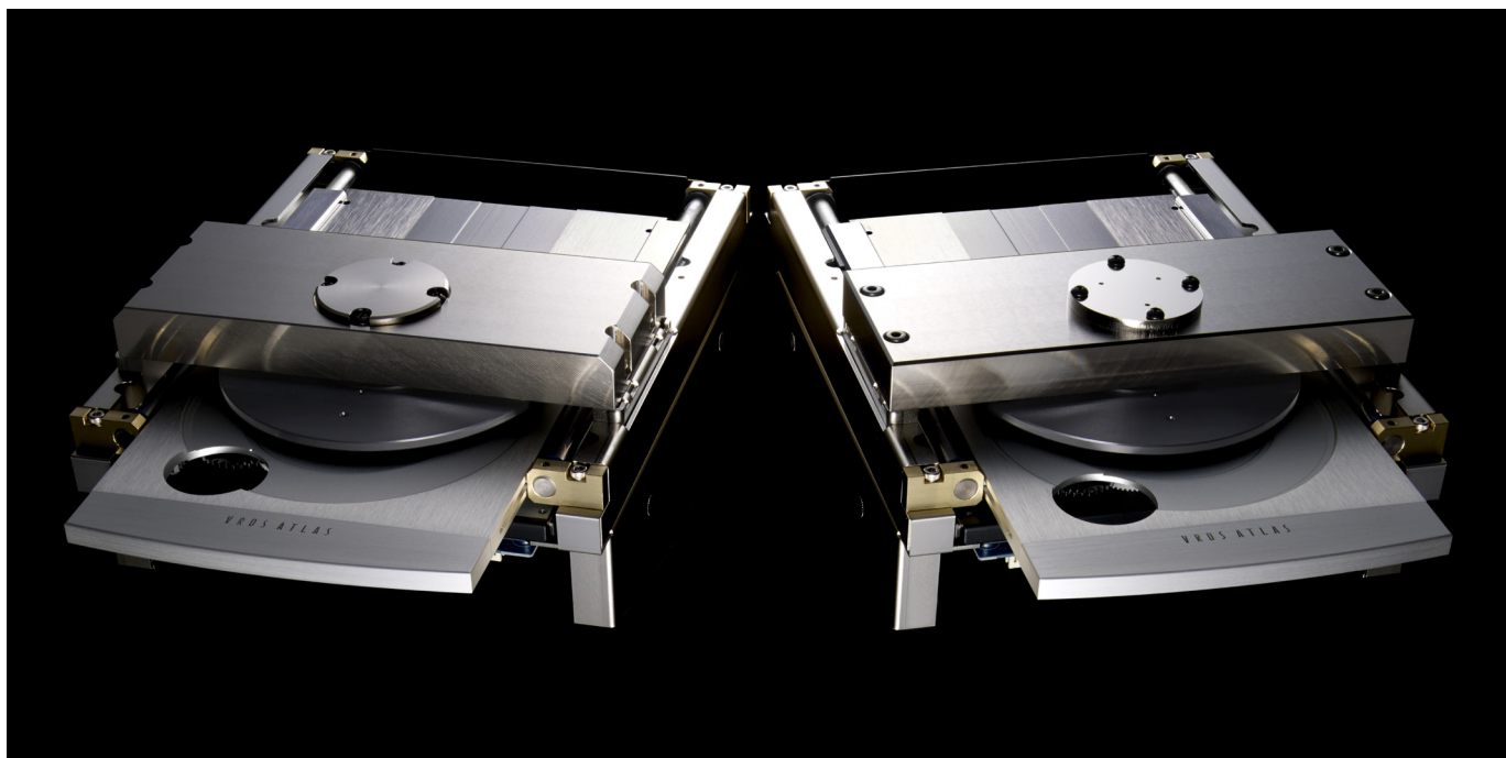
這就是Esoteric最新的VRDS-ATLAS 01雷射讀取系統，跟Grandioso系列所使用者一模一樣，只是二側板的厚度稍微薄些。
