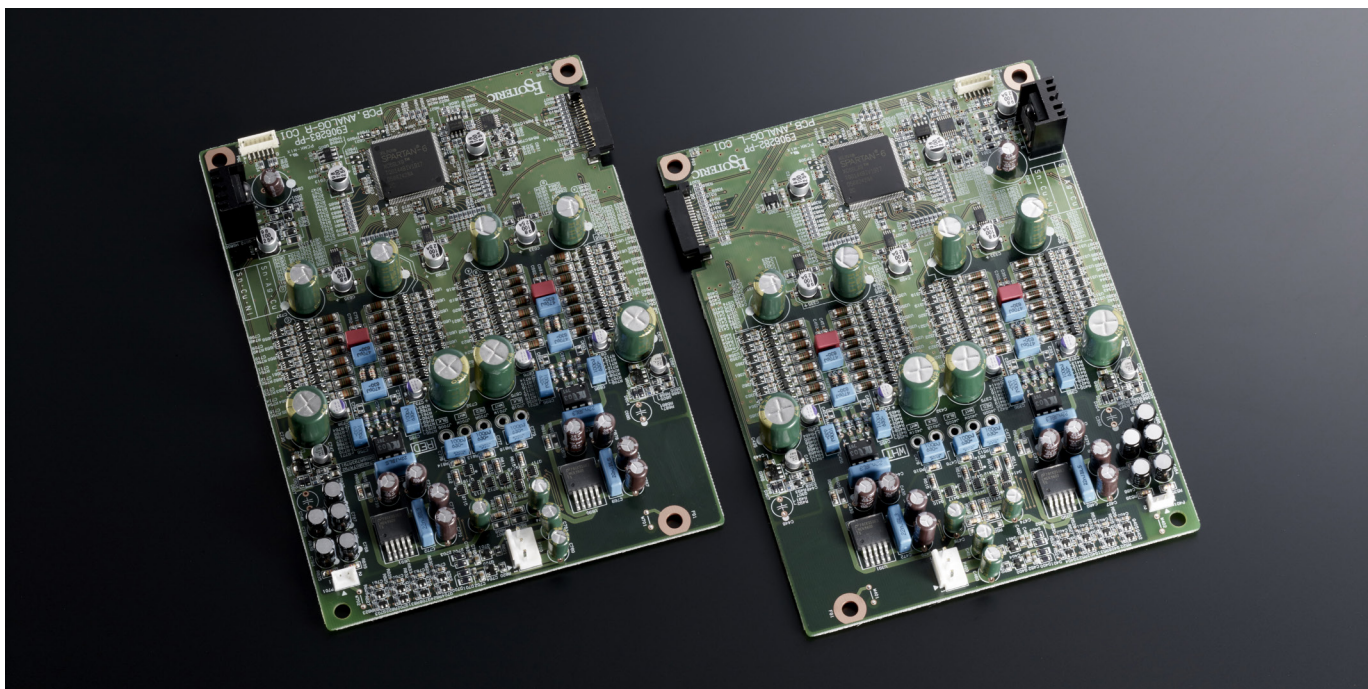
這是Esoteric最新的Master Sound Discrete DAC，與Grandioso D1X不同的是，K-01XD採用正常排列，而D1X因為空間足夠，採用圓形排列。
