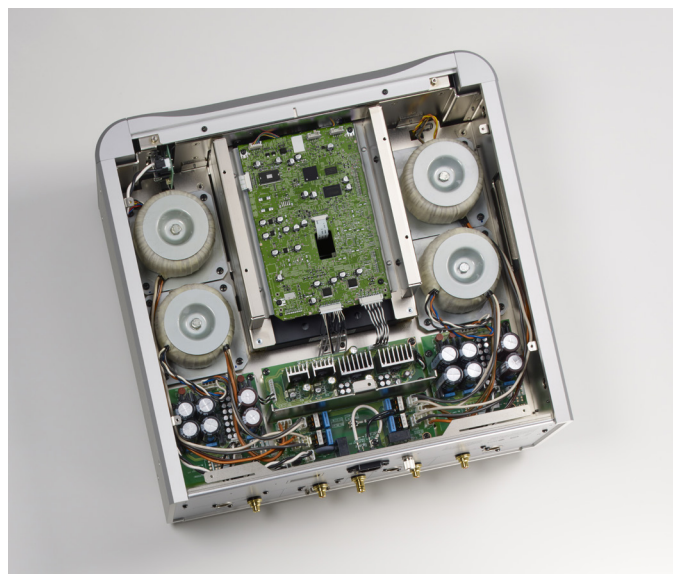
K-01XD的下層是電源供應，可以看到四個環形變壓器，以及電源濾波穩壓線路，負責供應不同的線路。
