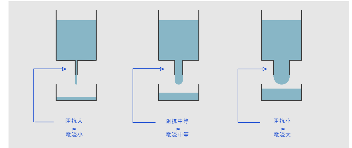
圖.3 具有相同水位或壓力 (=電壓) 的水箱
