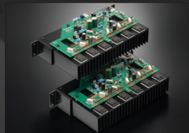
兼具通透感與立體音場的 30W 純 A 類功率放大模組
